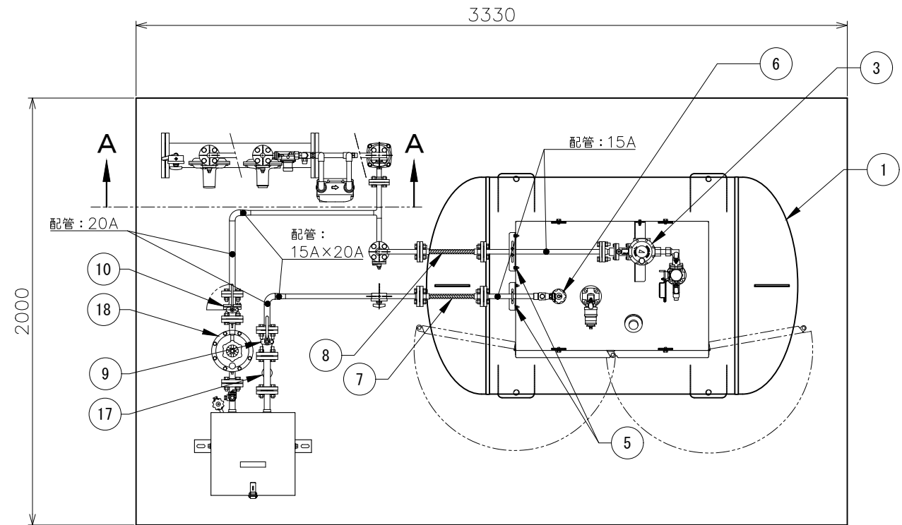
平面図
