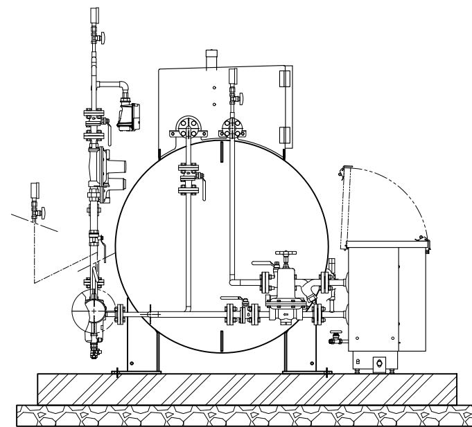
左側面図
