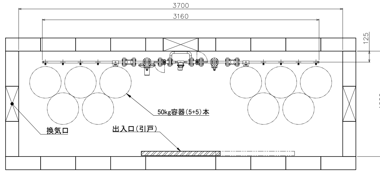
平面図
