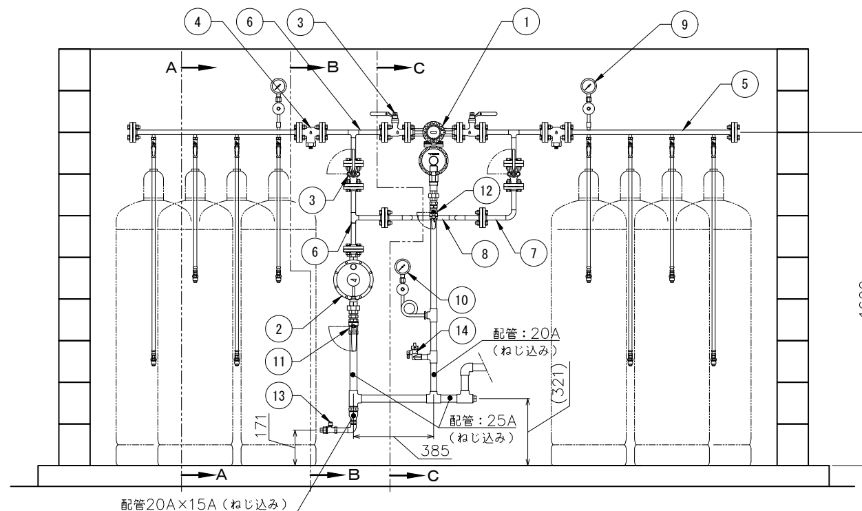
正面図
