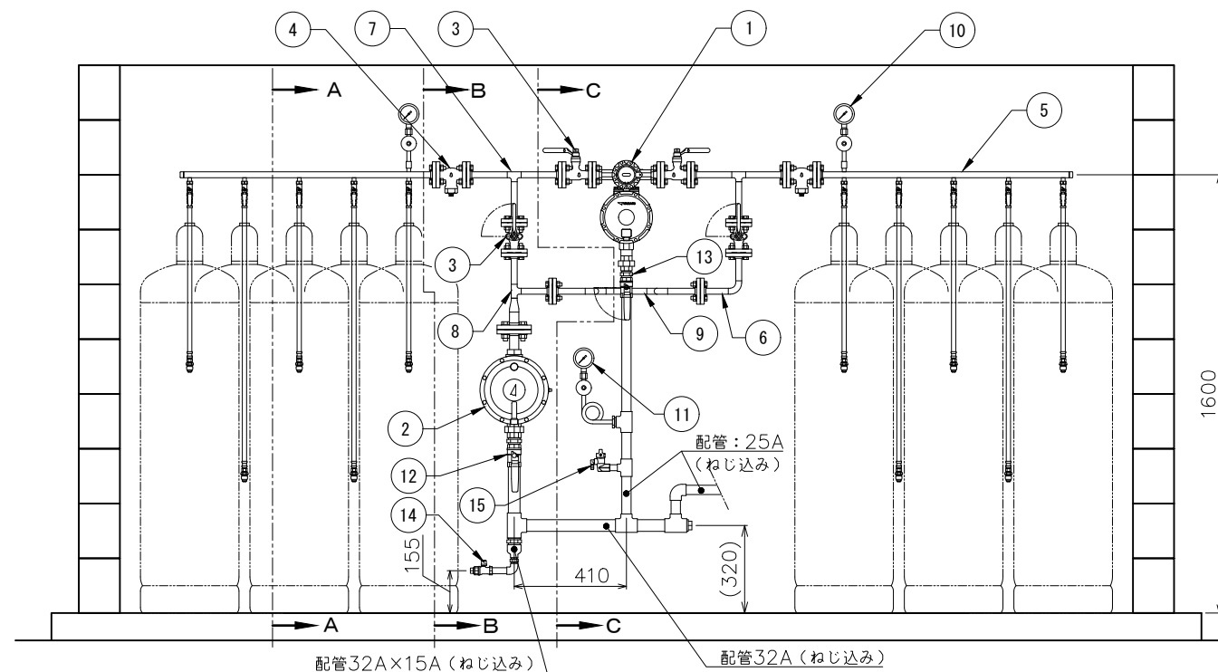
正面図
