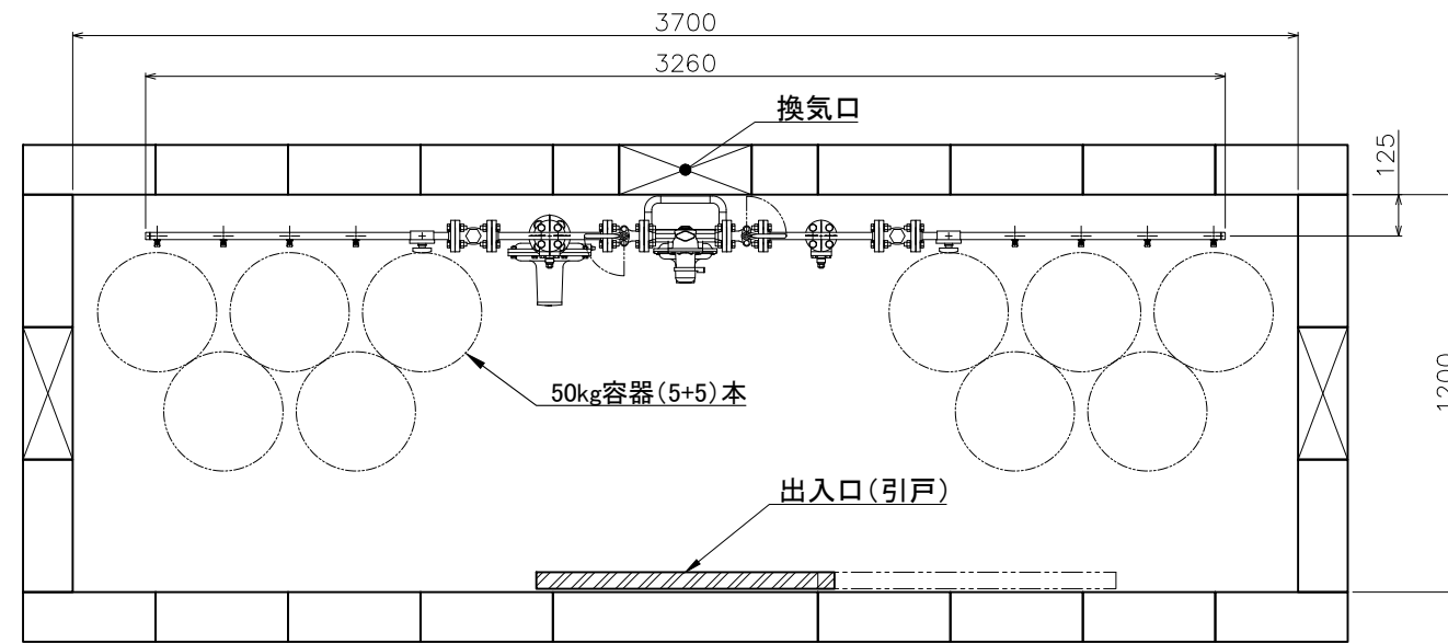
平面図
