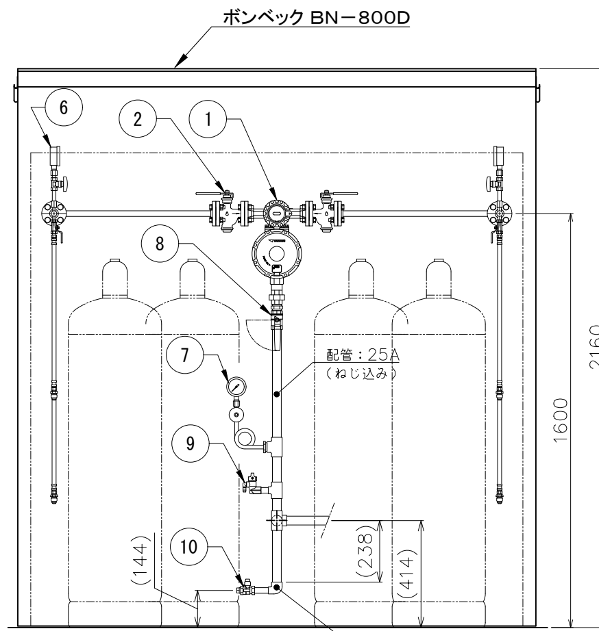
B-B (正面図)
