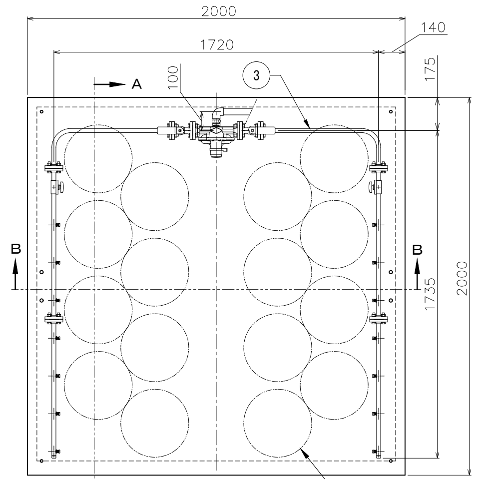
平面図
