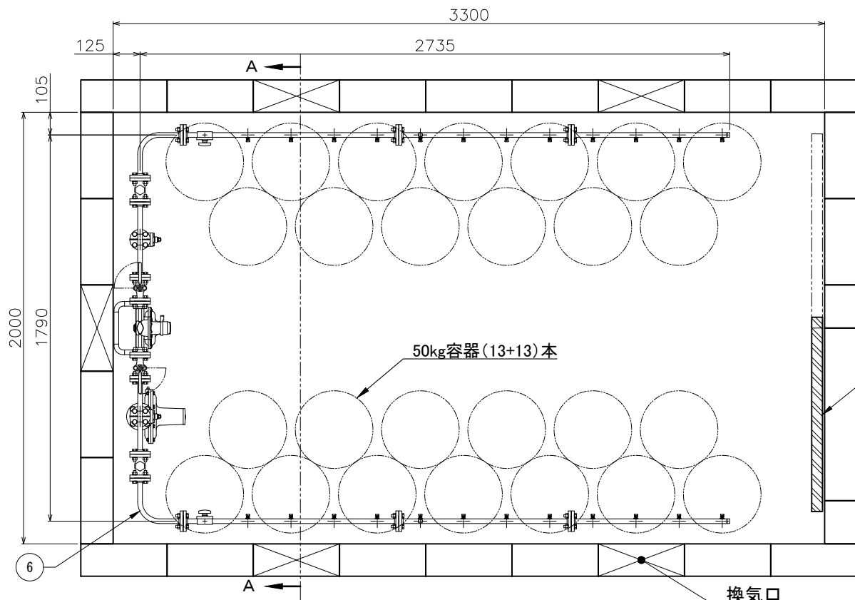
平面図
