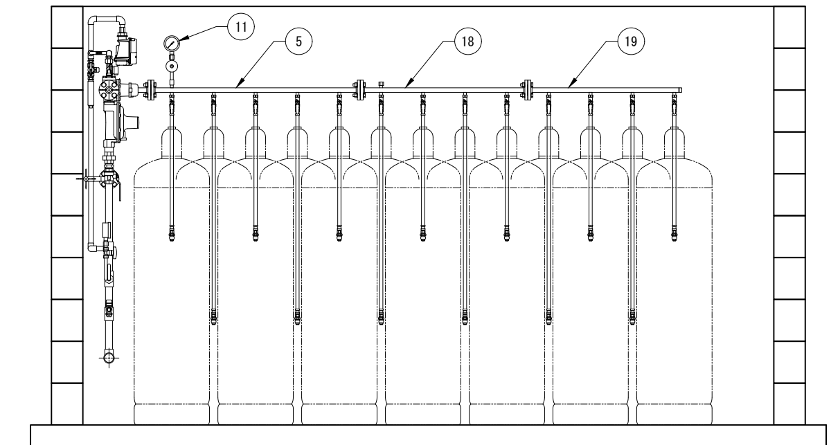
B-B
