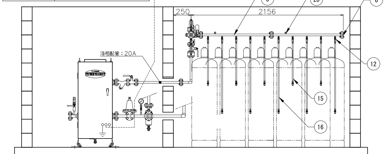
A-A (液相配管)
