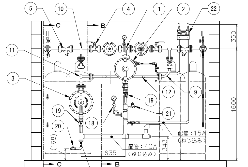
A-A (正面図)
