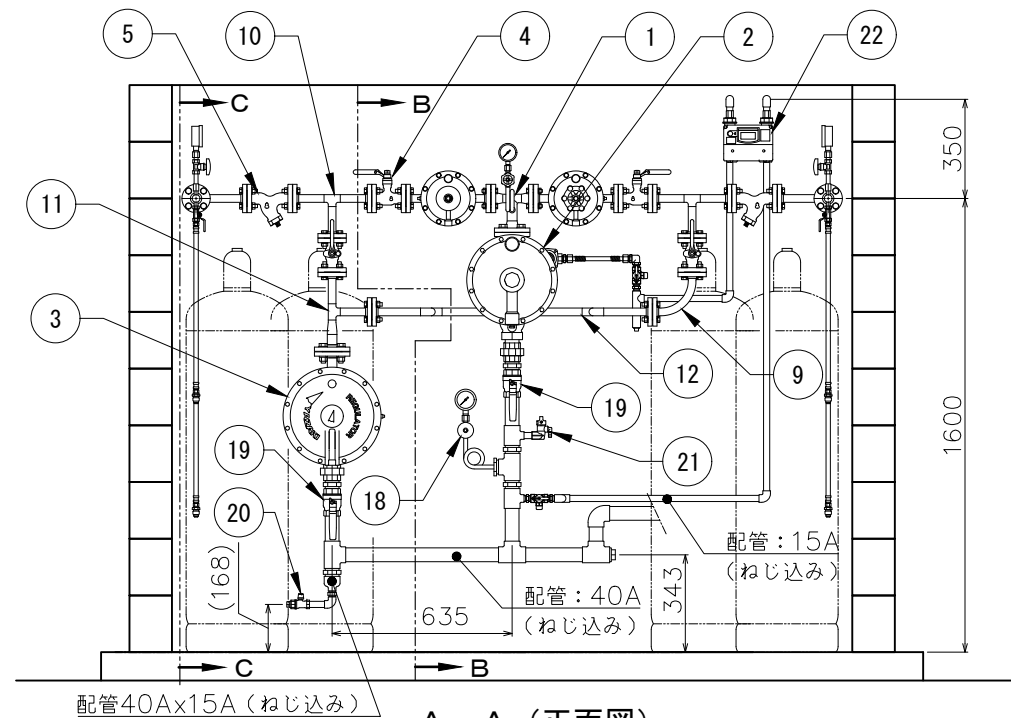
A-A (正面図)
