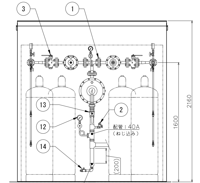
B-B (正面図)
