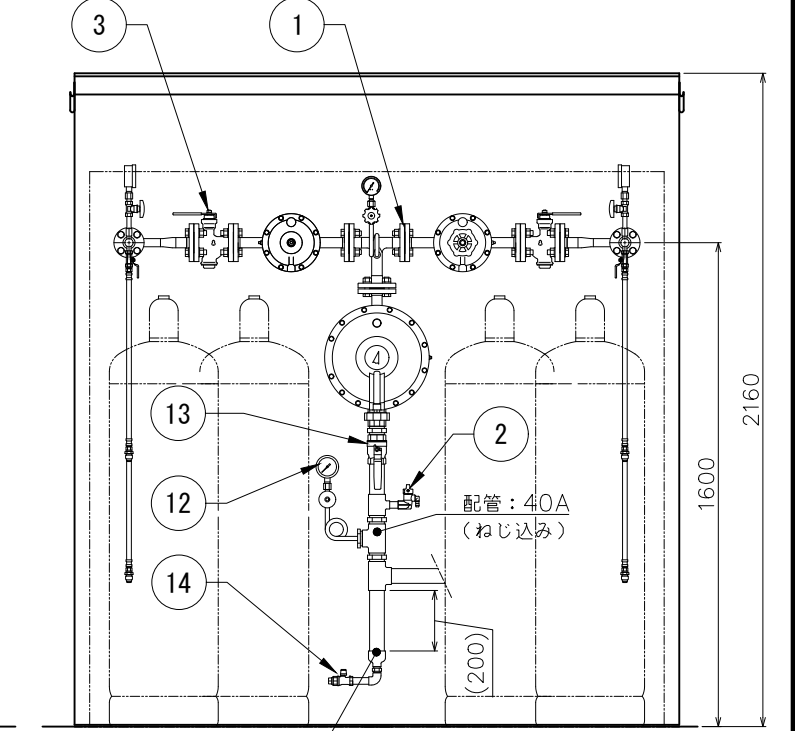
配管40Ax15A (ねじ込み) B-B (正面図)
