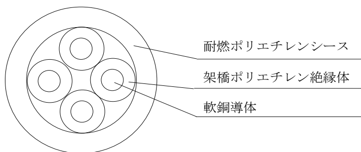
断面図
