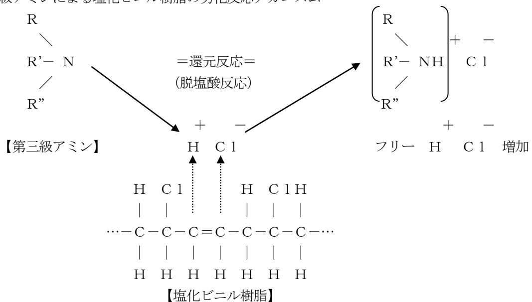
図-1 脱塩酸反応のモデル
